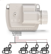
BL-IP1 (1 estación)
