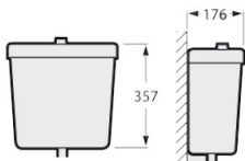
044102 TANQUE BAJO C/TAPA Y MECANIS. LATERAL POLO
