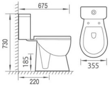
044099 INODORO T.ALTO S/VERTICAL VENECIA
