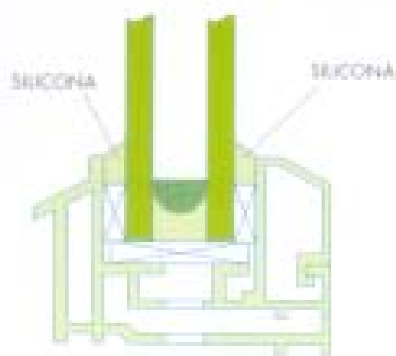
Juntas entre marco y vidrio
