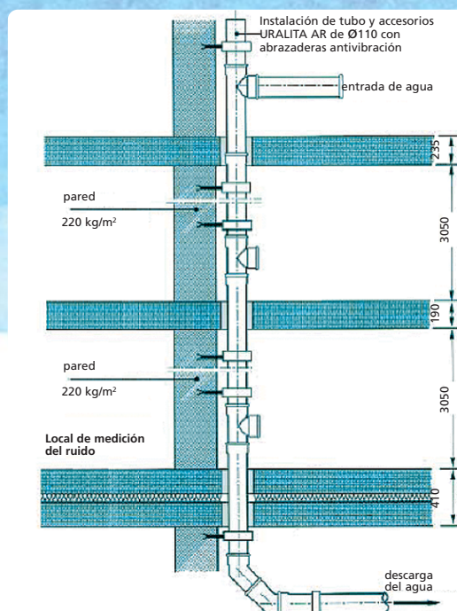
Esquema de instalación y local de medición del ruido, según norma UNE EN 14366. Ensayo realizado por el Fraunhofer Institut für Bauphysik de Stuttgart.
